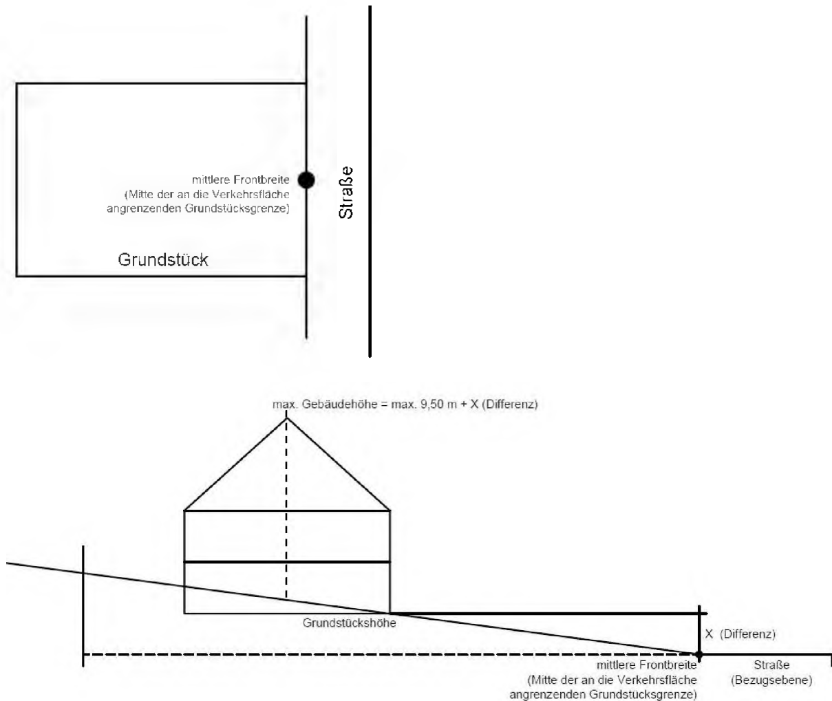
Abb.: Prinzipskizze zur Ermittlung der zulässigen Gebäudehöhe
